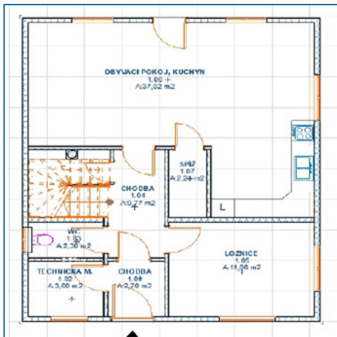
PŮDORYS 1.NP
