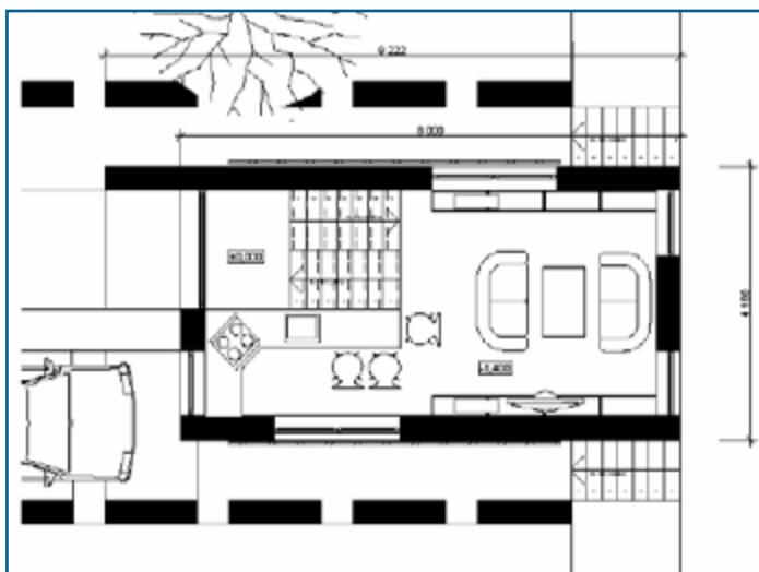
PŮDORYS 1.NP
