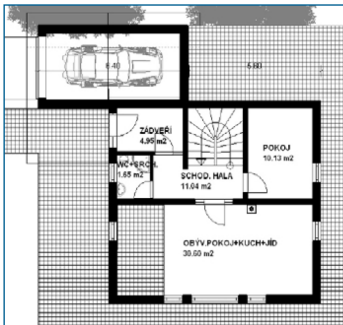
PŮDORYS 1.NP
