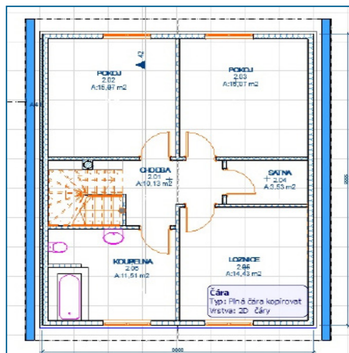
PŮDORYS 2.NP
